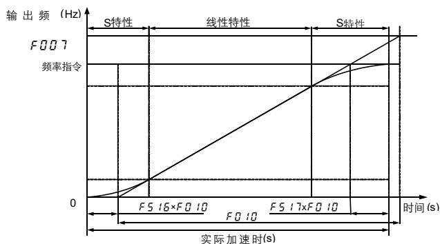
图 6.28 S 型曲线 1
