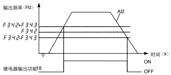
图 6.16 继电器输出-AI2 输入检出示意图
