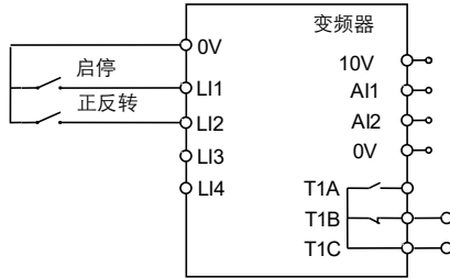
图 5.12 2 线控制模式 2-自锁开关正反转控制接线示意图
