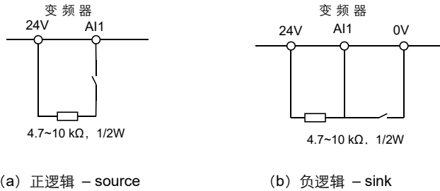
图 4.8 AI1 配置为逻辑输入端子时的接线图
