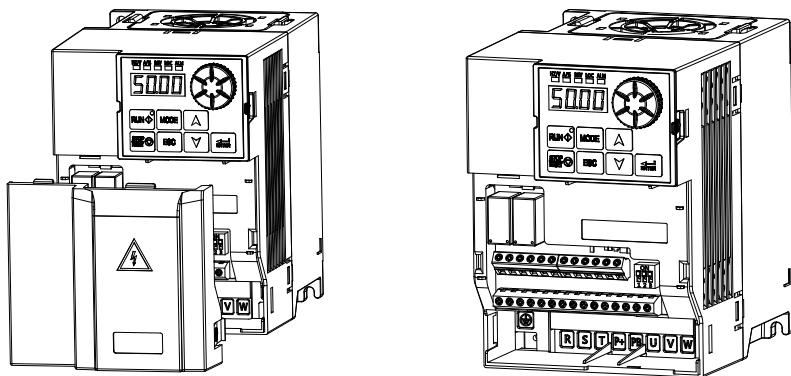
图 4.4 盖板、出线板的拆卸示意图
