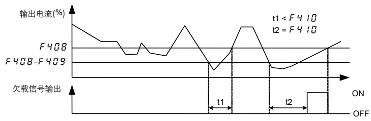
图 6.21 欠载信号输出示意图
