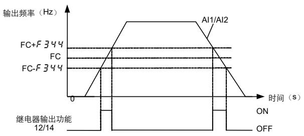
图 6.17 继电器输出-AI1 输入检出示意图
