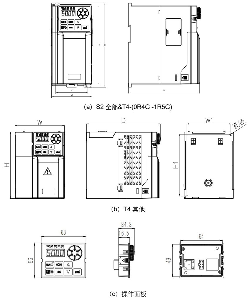
图 3.3 外形与安装尺寸
